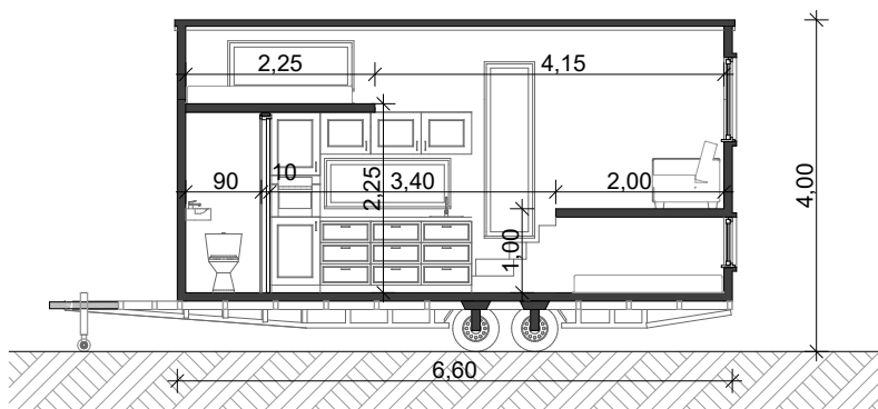
Hosszmetszet
