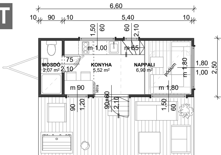
Földszint
