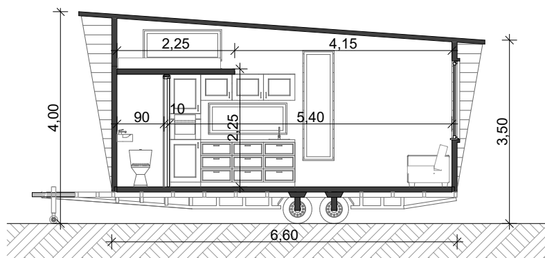
Hosszmetszet
