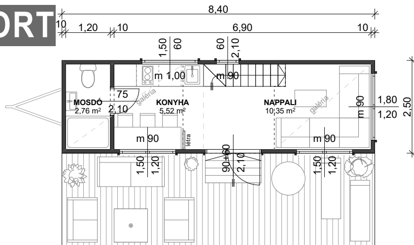
Földszint
