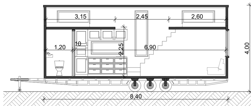
Hosszmetszet
