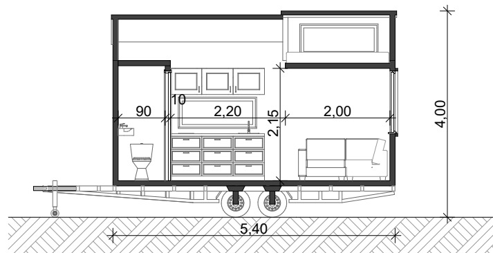
Hosszmetszet
