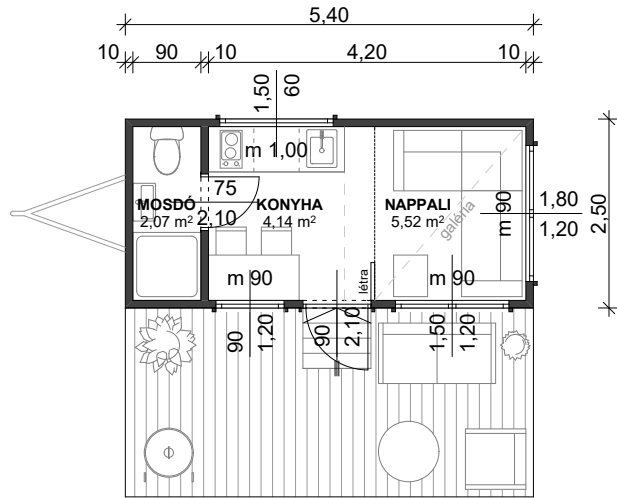
Földszint
