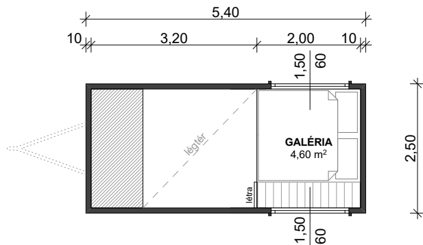
Galéria
